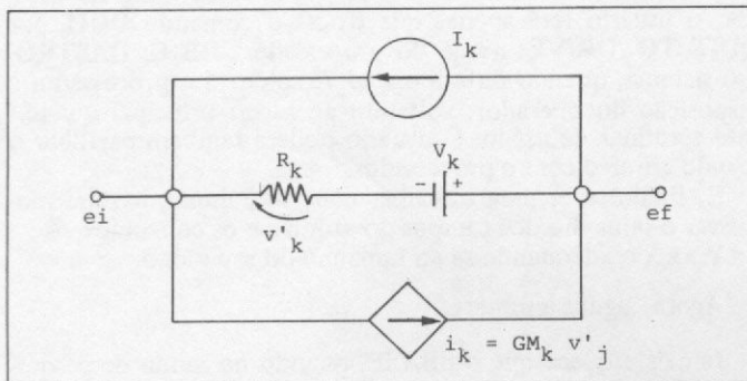
Figura 1 – Ramo genérico k com nó inicial i e nó final f
